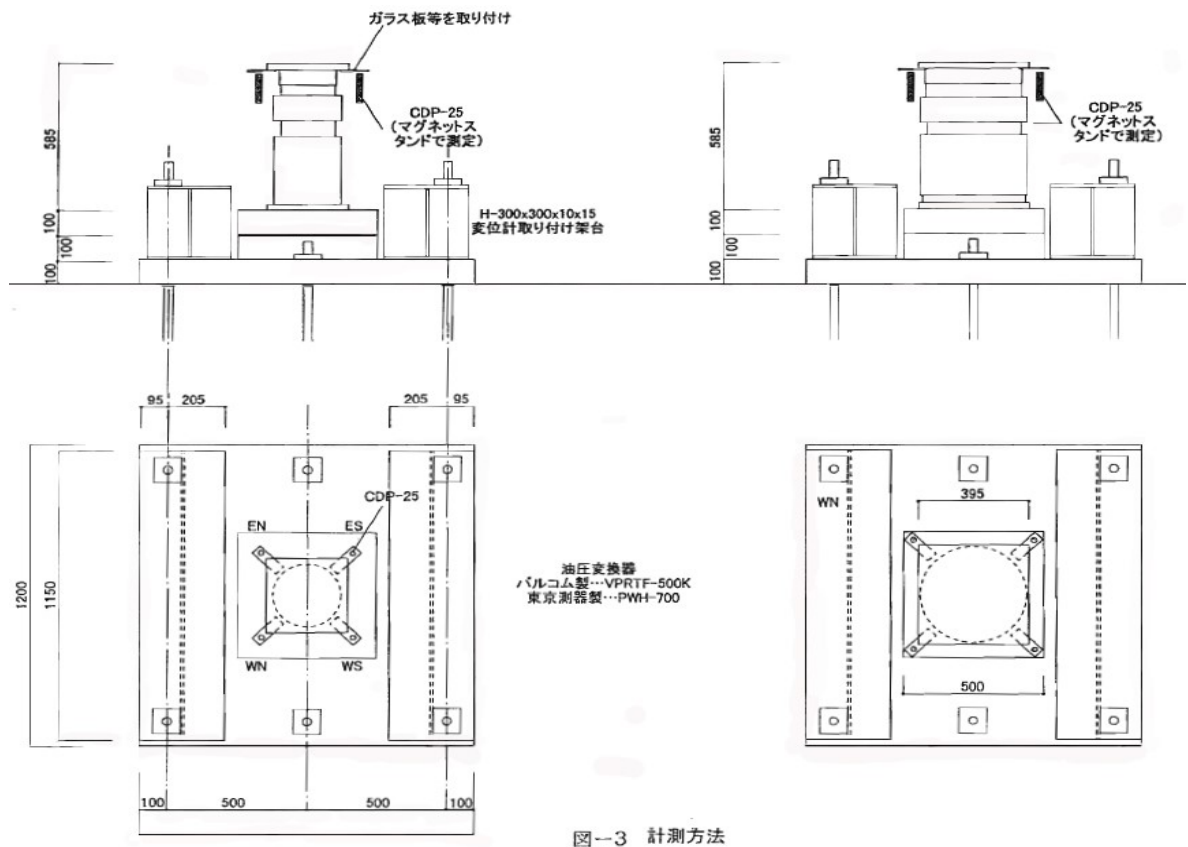
図-3 計測方法
