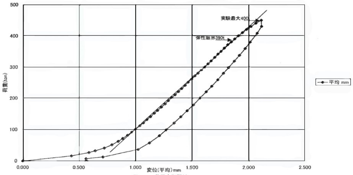
圖4-d 荷重変形關係
