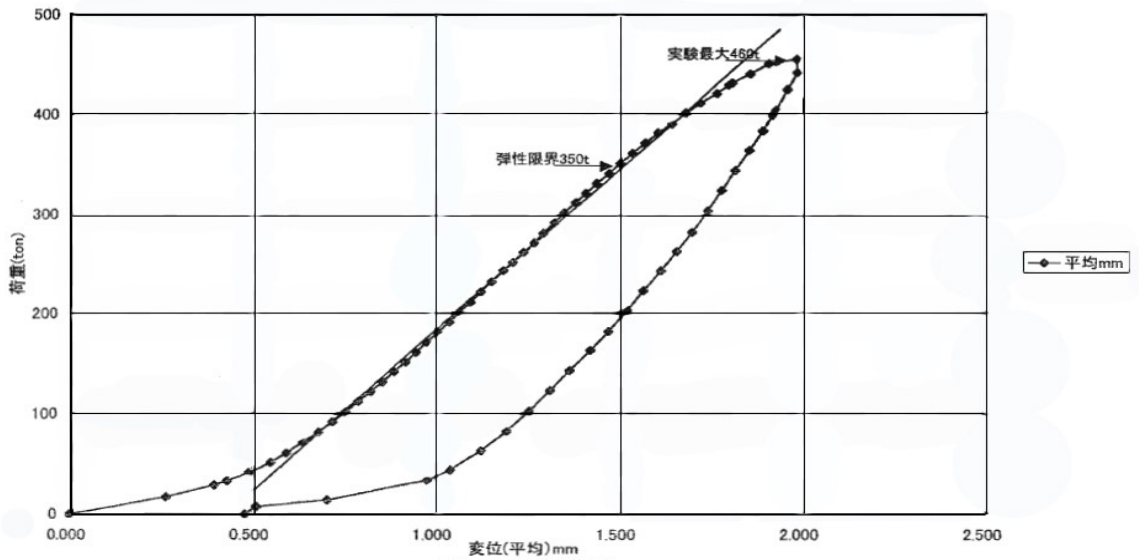
圖4-e 荷重変形關係
