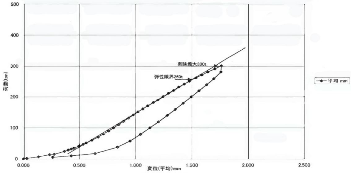
圖4-b 荷重変形關係
