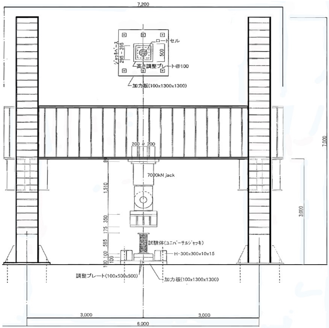
図-2 荷装置置図 S: 1/50
